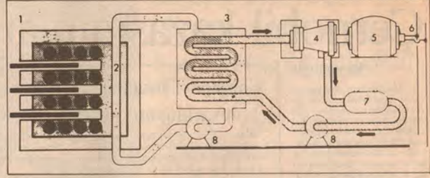
1- Reaktör 2- Isı enerjisinin komple derece soğutma su sistemi ile nakli 3- Reaktörden gelen suyun ısıtım ikinci bir soğutucu sisteme devrini sağlayan radyatör, 4- Türbin 5- Jeneratör 6- Elektrik hattı 7- Türbinden gelen buharın su haline dönüştüğü soğutucu 8- Su pompaları.
