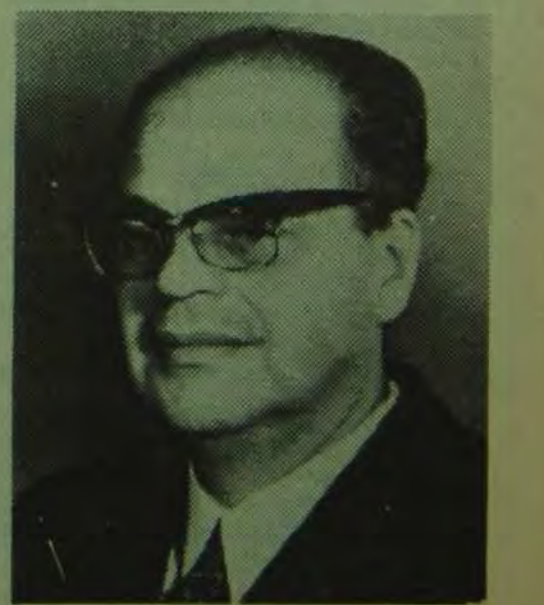
Nikolay Basov: Lazeri bulan üç fizikçiden biri (SSCB).
