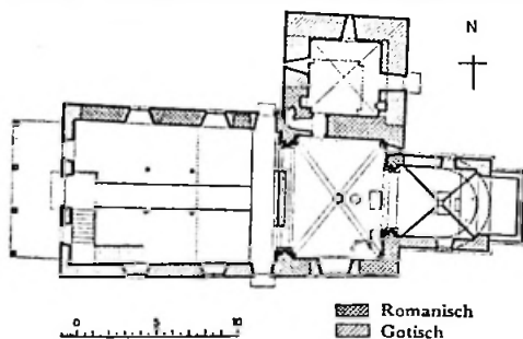
Grundriß der Kirche. Maßstab 1:500
