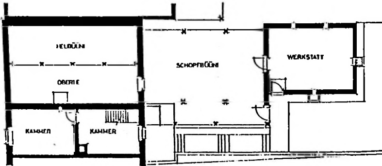
Obergeschoss
