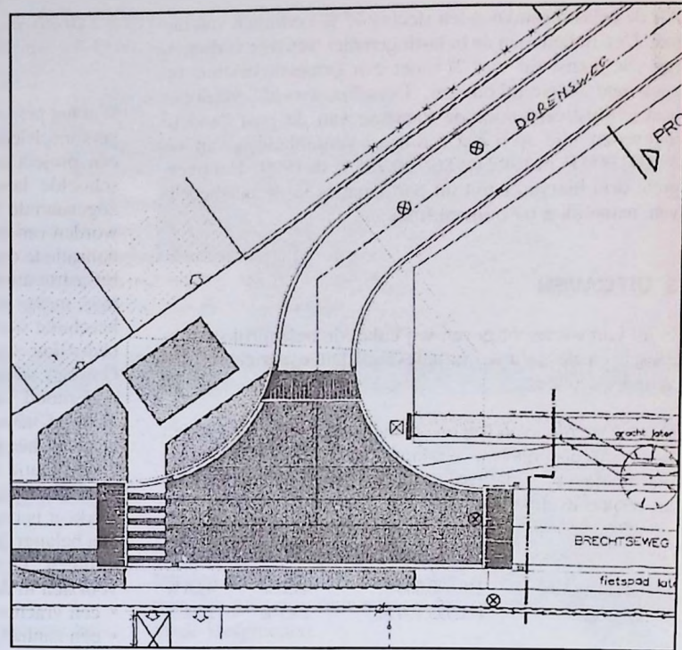
De aansluiting Dorensweg - Brechtseweg met een verkeersplateau
