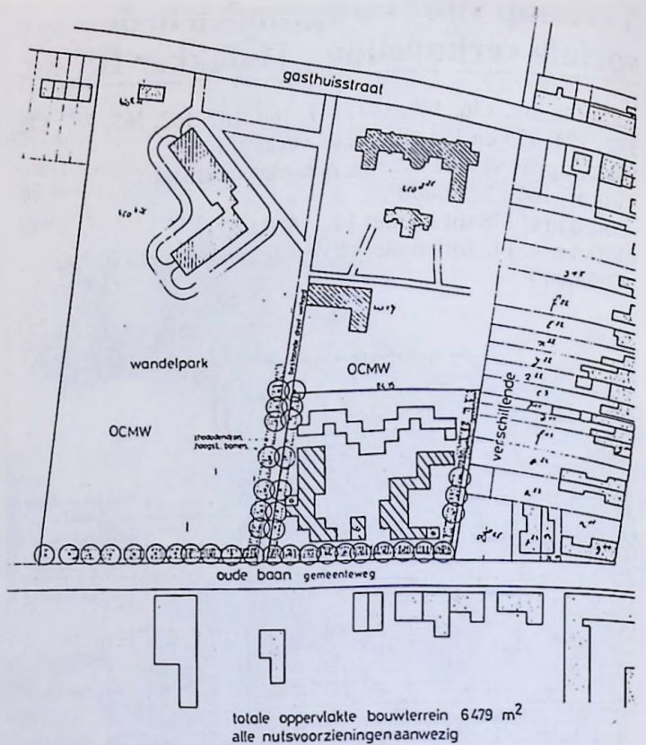
liggingsplan 1/1000 Plan van het project voor de 14 bejaardenwoningen.
