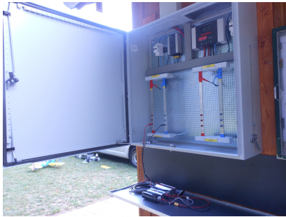
Blick ins Innenleben mit Elektronik
