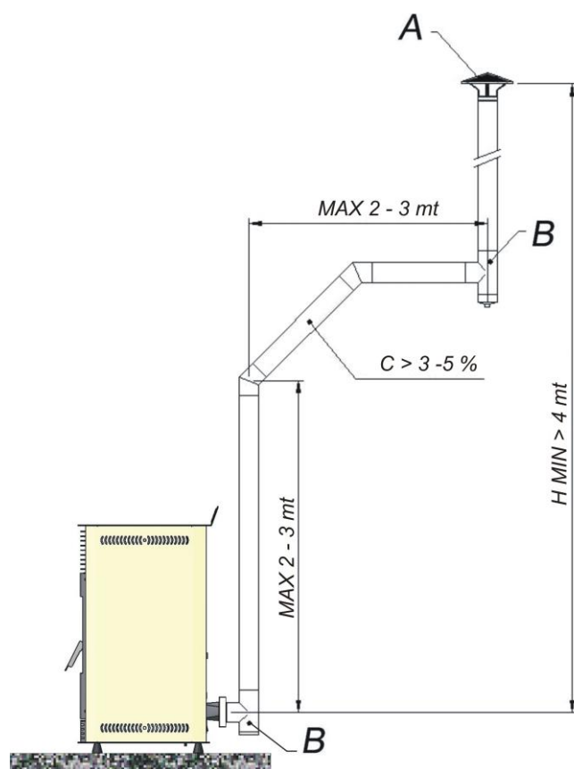
Esquema de instalação de saída de humos (fig. 2)
