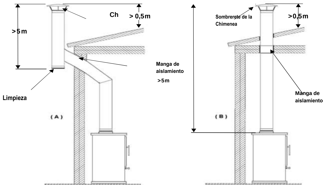
Figura 2. Ejemplo de instalación de chimenea
